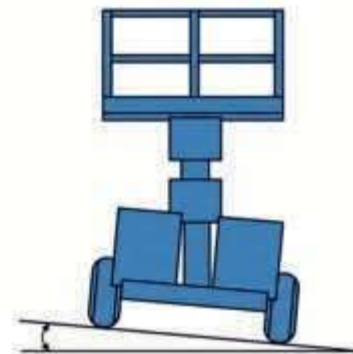
13° Maximaler Schiefstand
